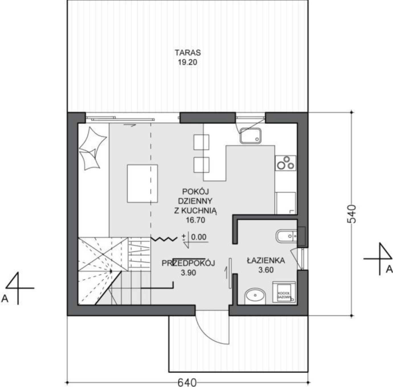
RZUT PARTERU
