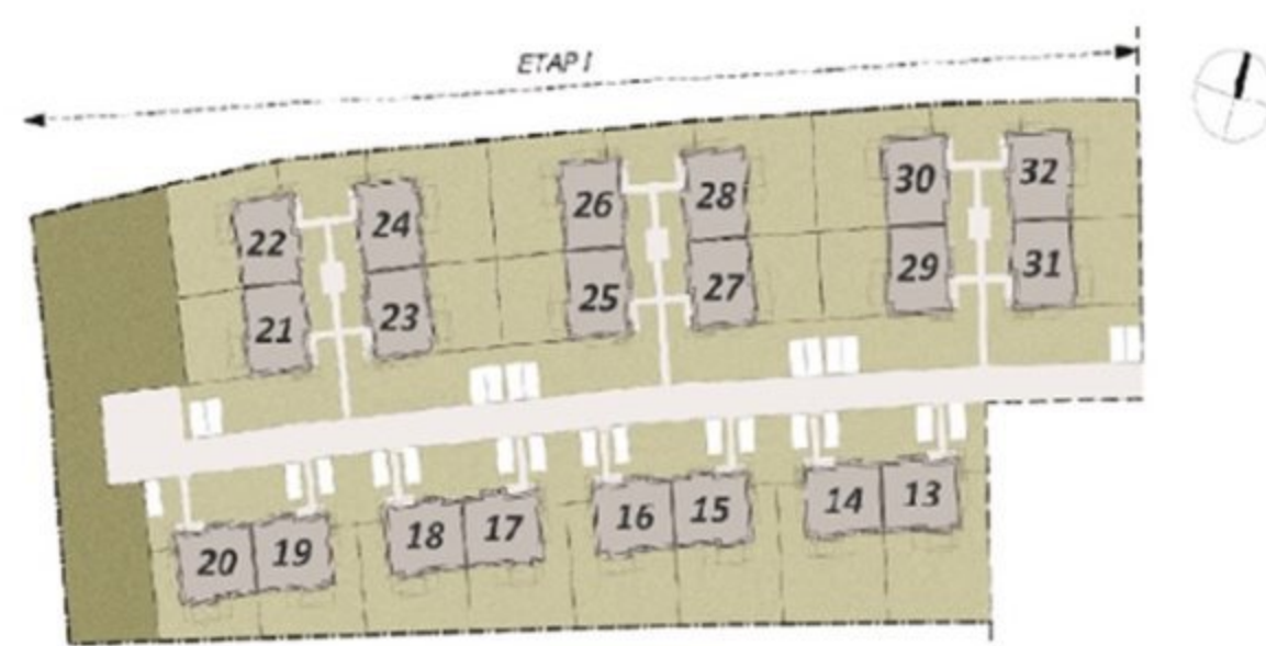
ZAGOSPODAROWANIE TERENU
