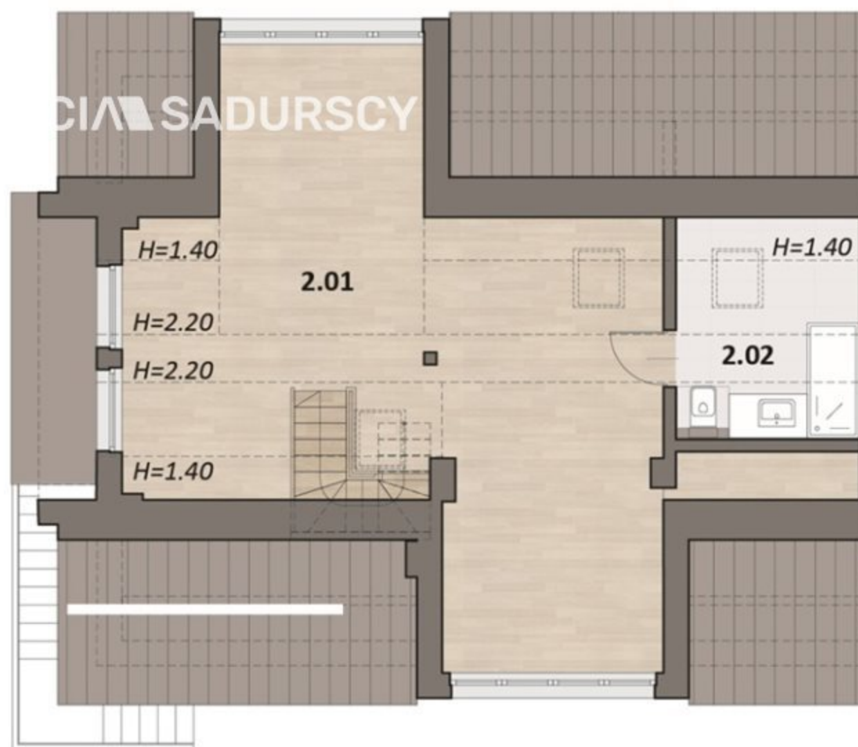
RZUT PODDASZA
