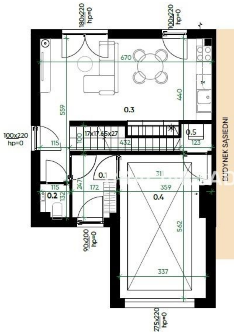
RZUT PARTERU
