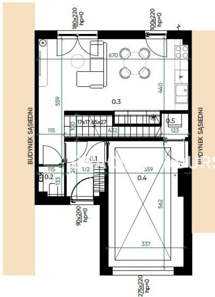
RZUT PARTERU
