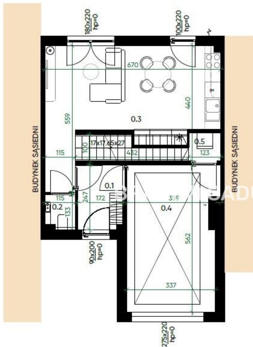
RZUT PARTERU
