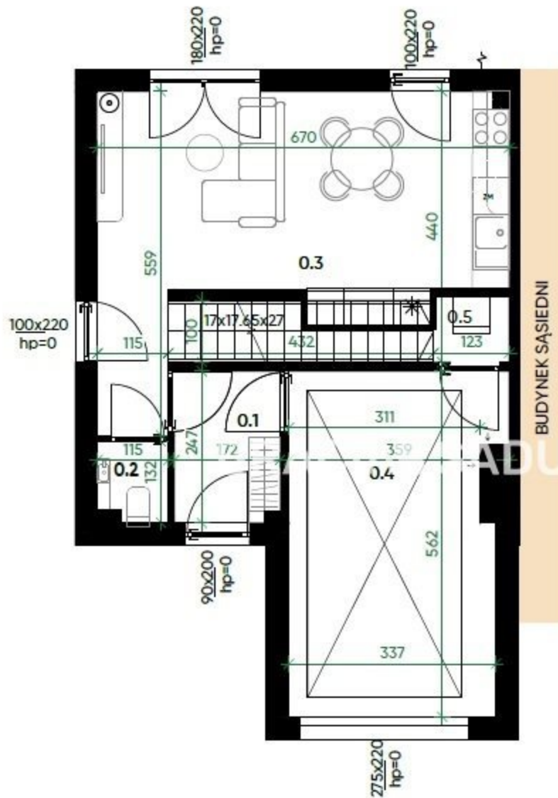
RZUT PARTERU
