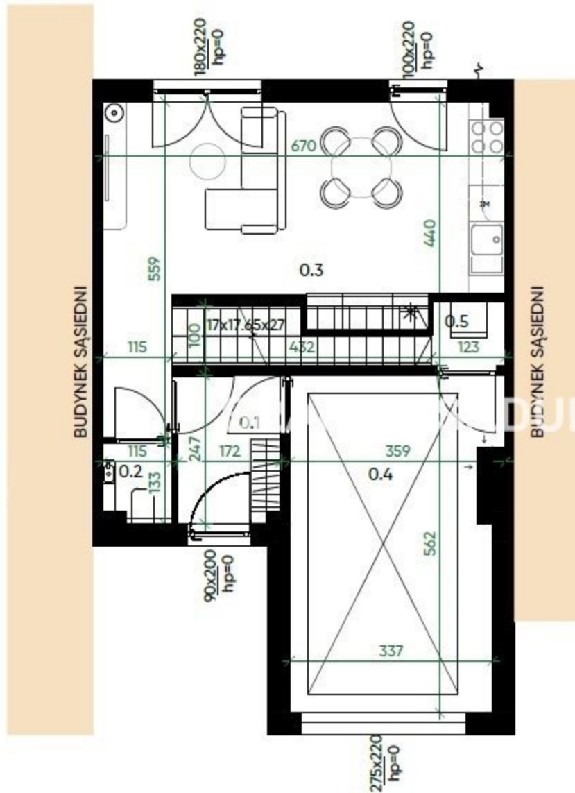
RZUT PARTERU
