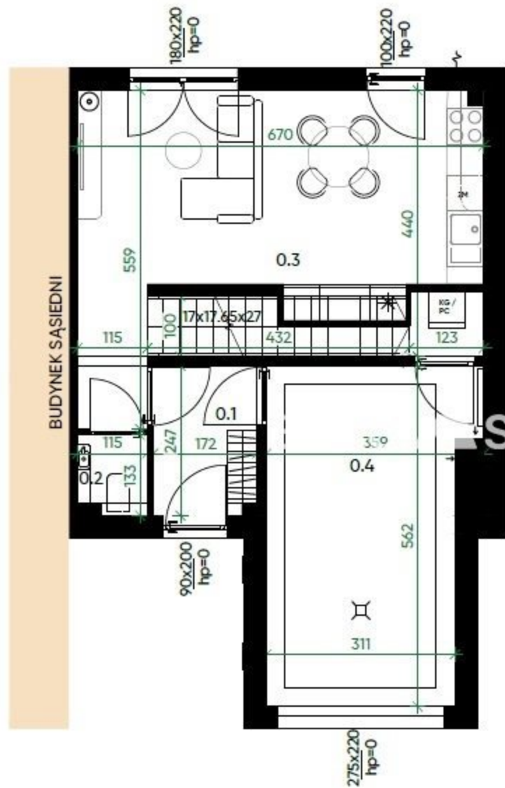
RZUT PARTERU
