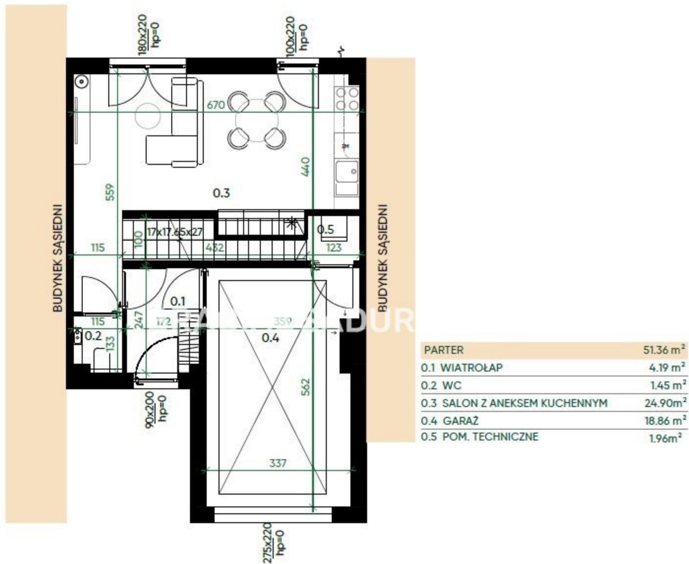
RZUT PARTERU
