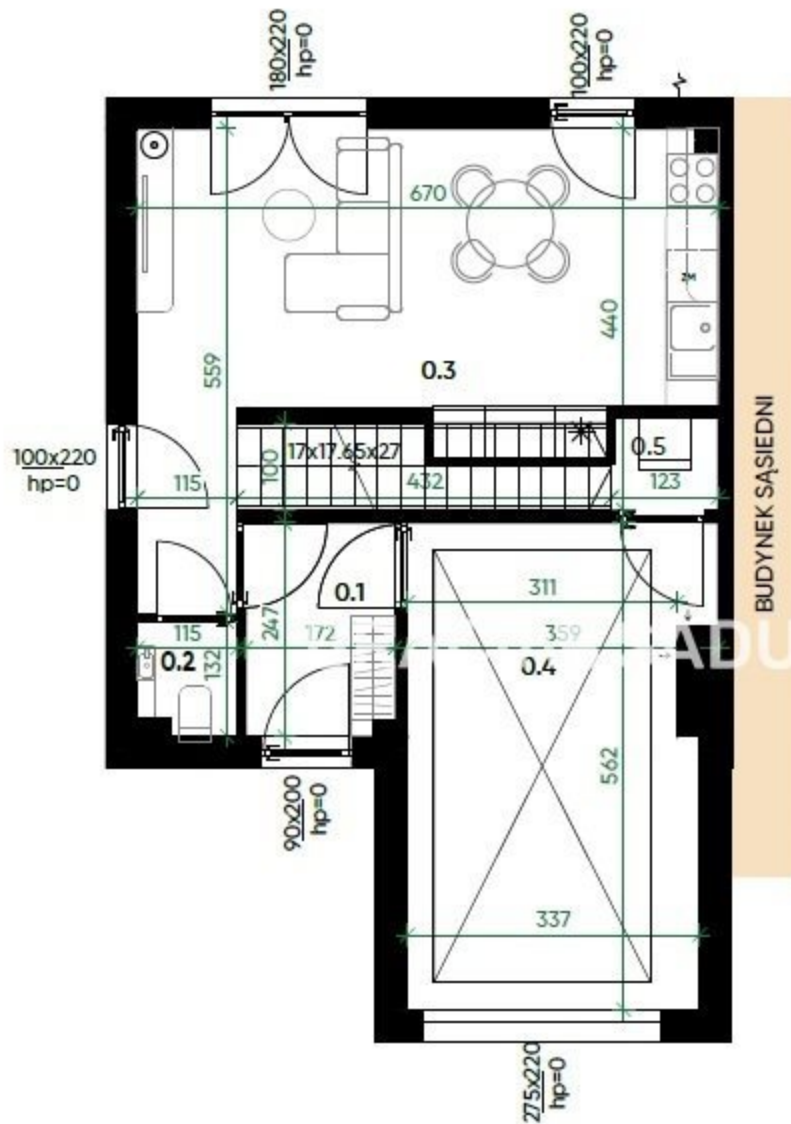
RZUT PARTERU
