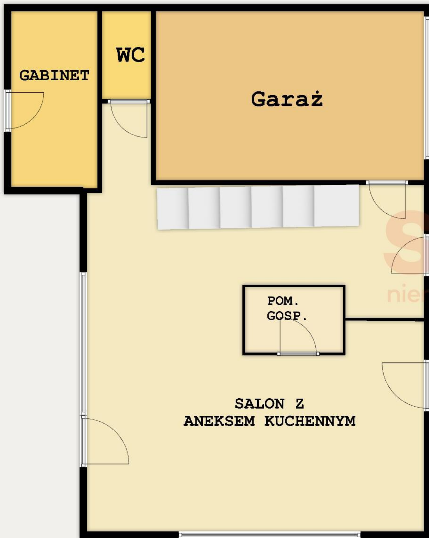
POZIOM 0
