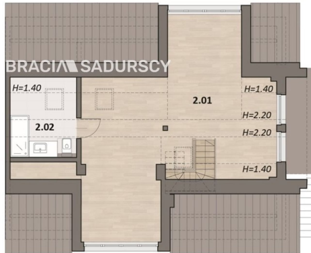
RZUT PODDASZA
