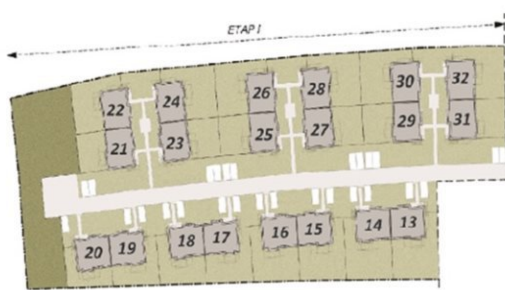
ZAGOSPODAROWANIE TERENU
