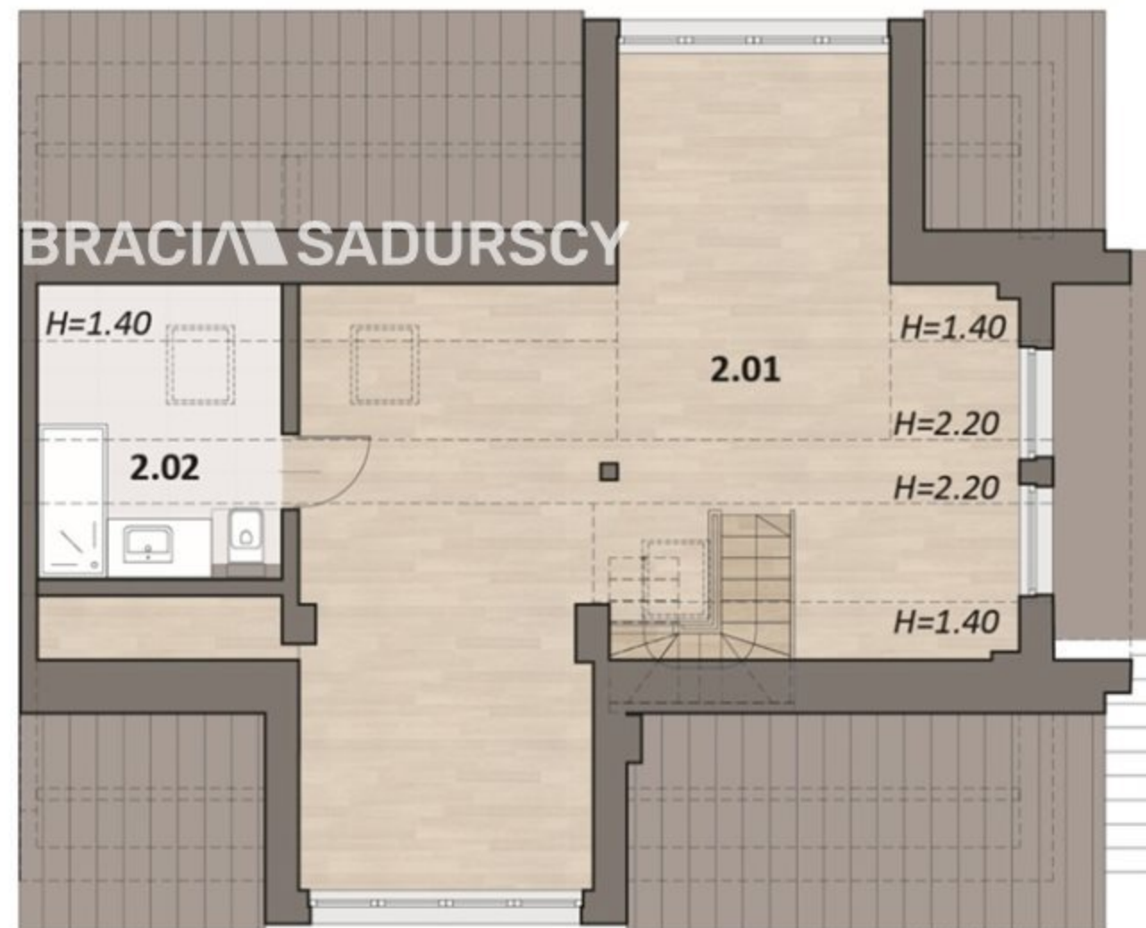
RZUT PODDASZA
