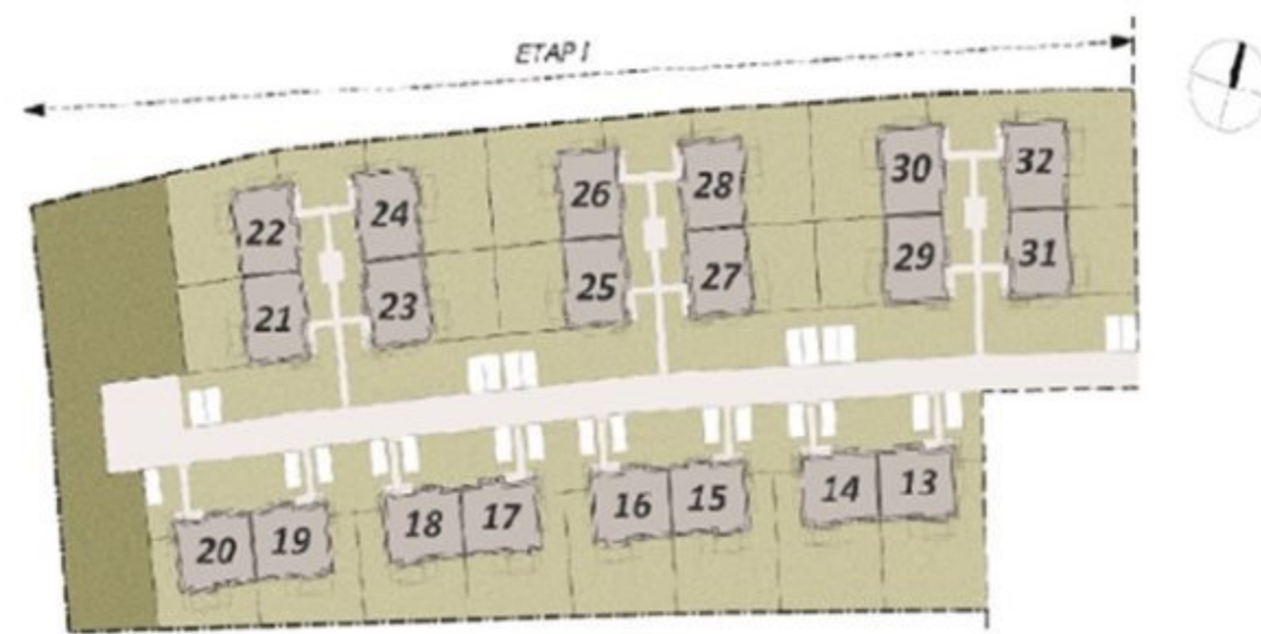
ZAGOSPODAROWANIE TERENU
