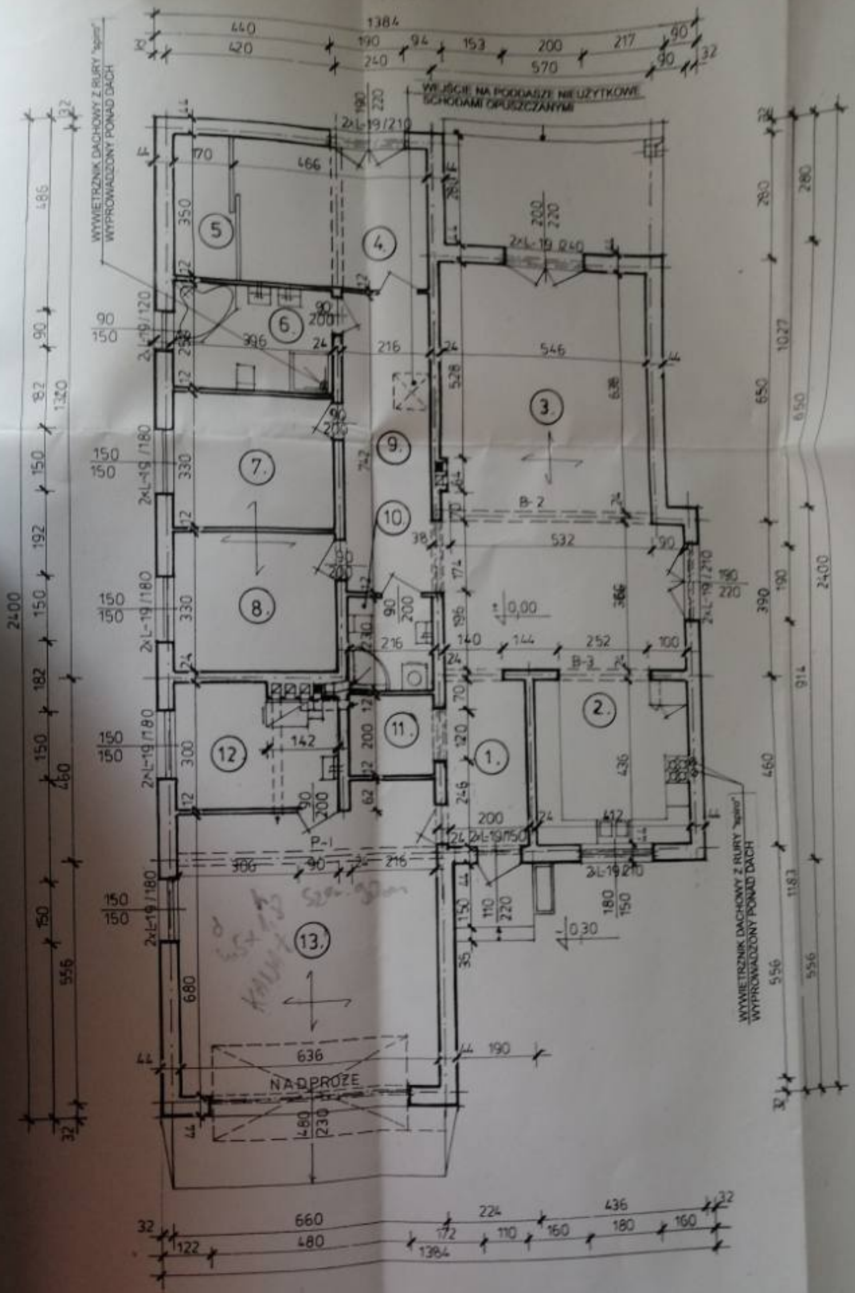
RZUT PARTERU 1 : 100
