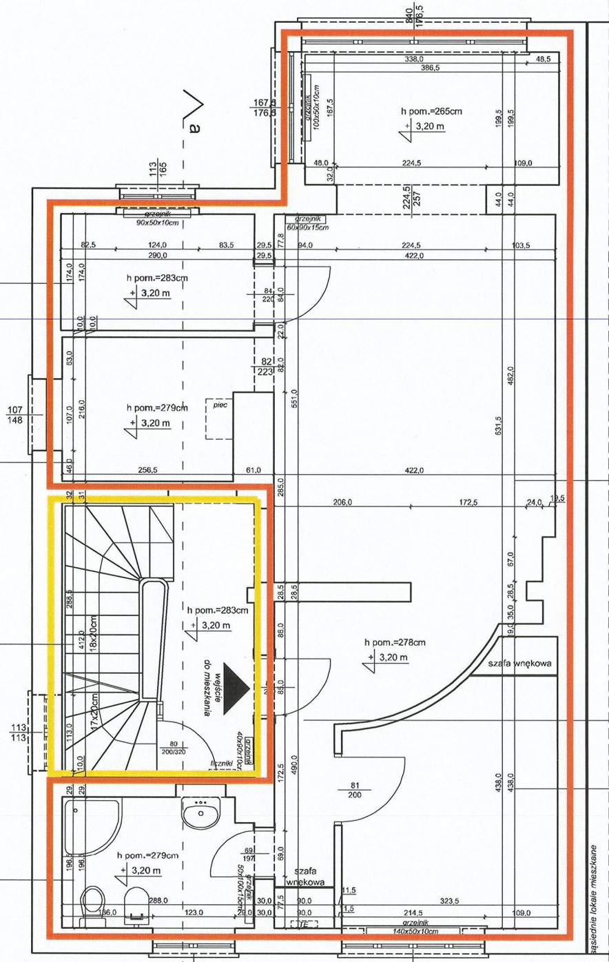
rzut poziomym +1
