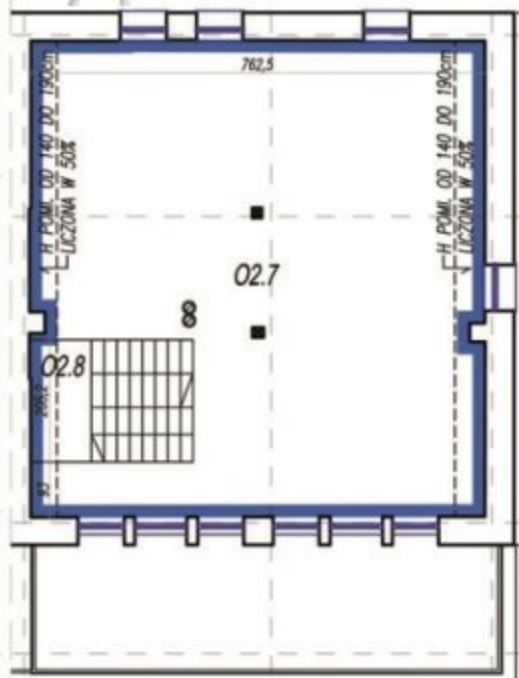
RZUT KONDYGNACJI TRZECIEJ NADZIEMNEJ
