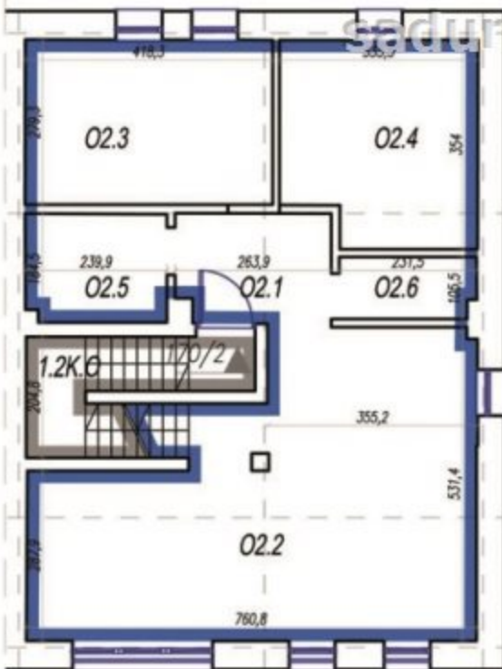
RZUT KONDYGNACJI DRUGIEJ NADZIEMNEJ
