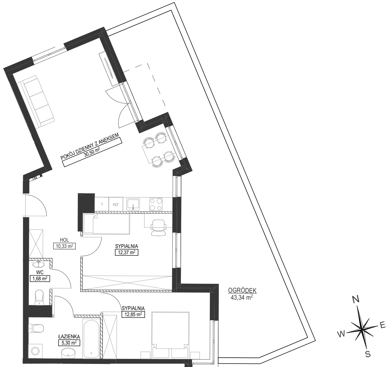
SCHEMAT LOKALU MIESZKALNEGO NA RZUCIE KONDYGNACJI
